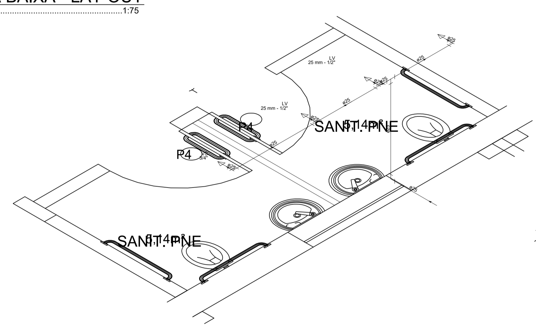
Detalhe H3 Escala 1:25
