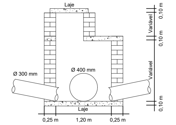
Detalhe dos Poços de Visita Sem Escala
